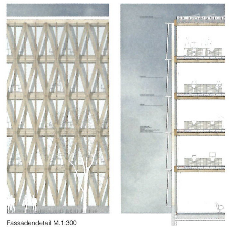
Fassadendetail M.1:300
