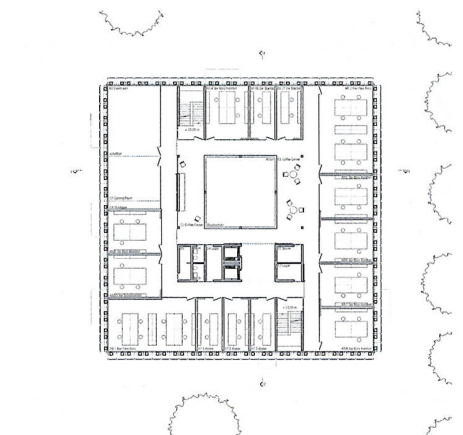
Grundriss 4. Obergeschoss M.1:750
