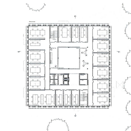
Grundriss 1. Obergeschoss M.1:750
