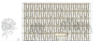
Ansicht Eingang M.1:750
